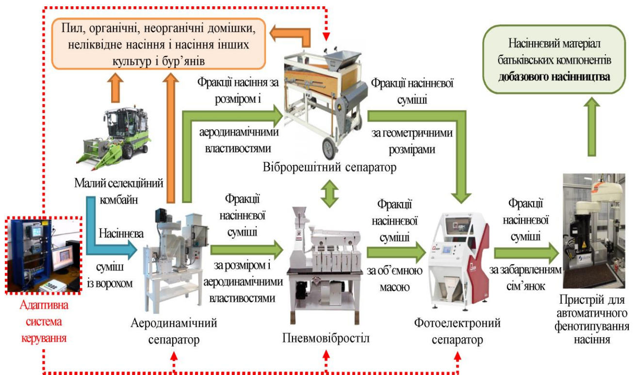
Рис. 3. Розроблена раціональна прецизійна технологічна лінія процесів сепарації насіннєвого матеріалу соняшнику для добазового насінництва
