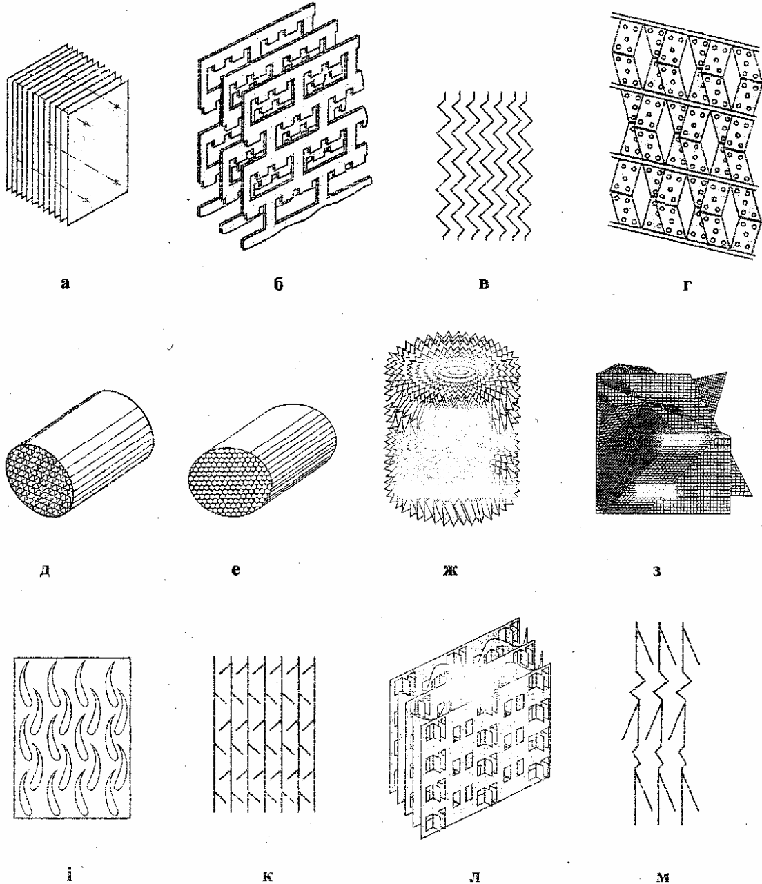
Рис.2. Основні типи регулярних пакетних насадок:
