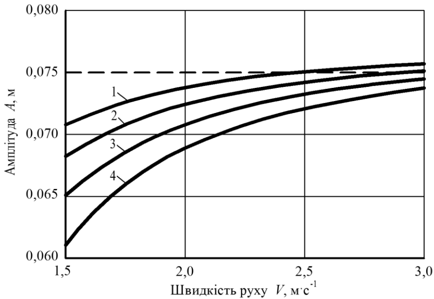
Рис. 4. – Залежність амплітуди A коливань ротора гичкозбиральної машини від швидкості V її руху при різному кроці нерівності поверхні ґрунту: 1 – l_1 = 0,6 м; 2 – l_1 = 0,7 м; 3 – l_1 = 0,8 м; 4 – l_1 = 0,9 м
