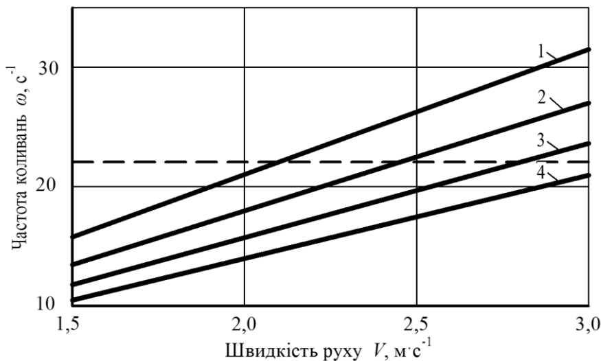
Рис. 5. – Залежність частоти \omega змушених коливань зрізано чого ротора у повздовжньо-вертикальній площині гичкозбиральної машини та швидкості V її руху при різному кроці нерівностей поверхні ґрунту: 1 – l_1 = 0,6 м; 2 – l_1 = 0,7 м; 3 – l_1 = 0,8 м; 4 – l_1 = 0,9 м
