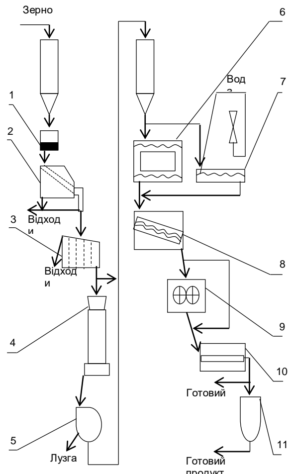
Рис. 1 Типова технологічна схема виробництва зернової мікронізованої продукції: 1 – магнітний захист; 2 – зерноочисний сепаратор; 3 – каменевідбірник; 4 – лушчильна машина; 5 – повітряний сепаратор; 6 – пропарювач; 7 – зволожувальна машина; 8 – мікронізатор; 9 – плушчильний верстат; 10 – охолоджувальна колонка горизонтального типу; 11 – дробарка
