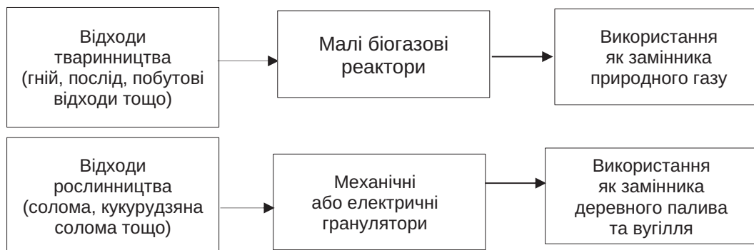
Рис. 1. Принципова схема переробки відходів сільськогосподарської діяльності в особистих селянських господарствах на біогаз та тверде біопаливо
