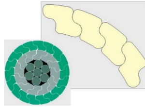
Рис. 4. Конструкція проводу AERO-Z
