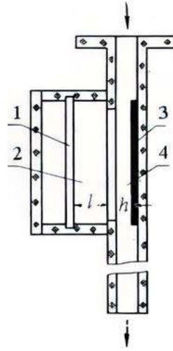
Рис. 1. Будава іонізаційної приставки: 1 – джерело \alpha -частинок; 2 – іонна камера; 3 – сепаруючий електрод; 4 – повітропровід
